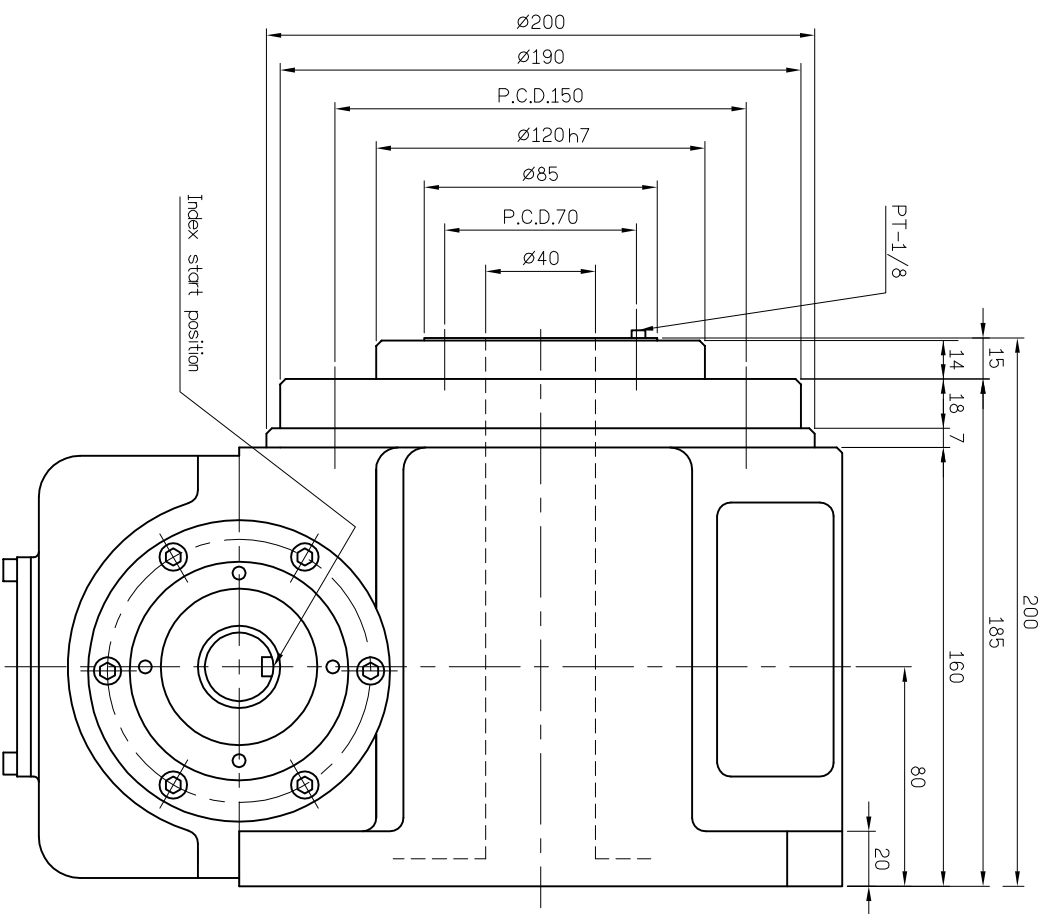
DT110D,外觀尺寸圖 110DT-OUT
